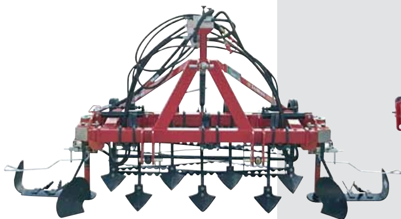
Καλλιεργητής B.T. SRF - 2A Cultivator "HEAVY-TYPE" SRF - 2A
