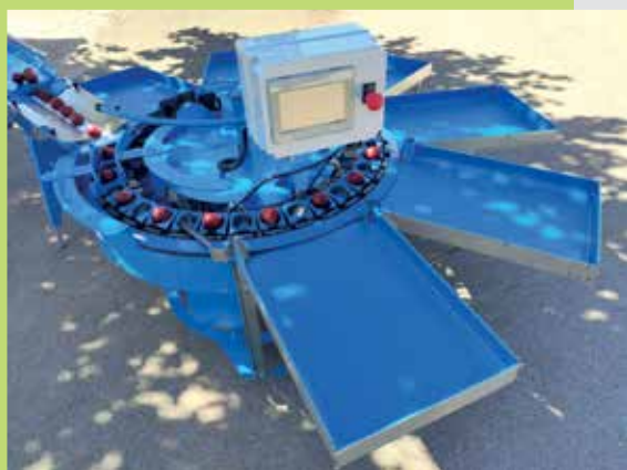
Διαλογητήριο CALIBREX: MINIGRAM 2(+) Grader CALIBREX: MINIGRAM 2(+)
